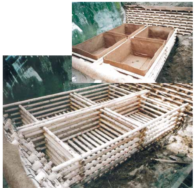
C-15 木製水叩工 杉・横木3.0m×φ10cm 杉・横木2.0m×φ10cm (君津市・鎌滝)
